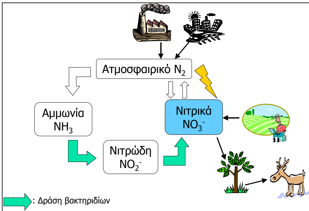
Εικόνα 2.5. Ο απλοποιημένος κύκλος του αζώτου.
